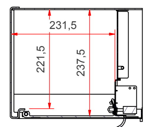
D-D (1:5)
