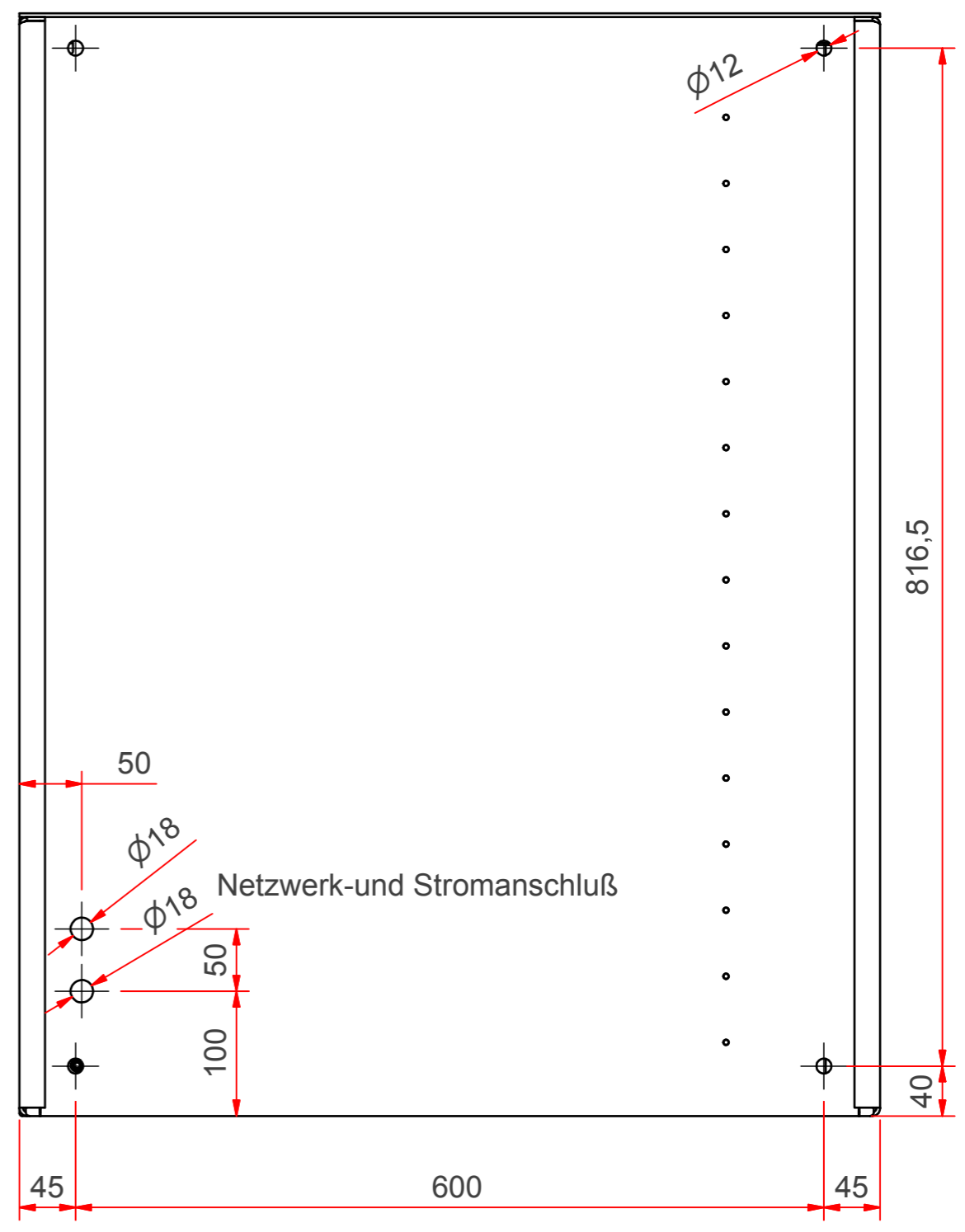
D-D (1:5)
