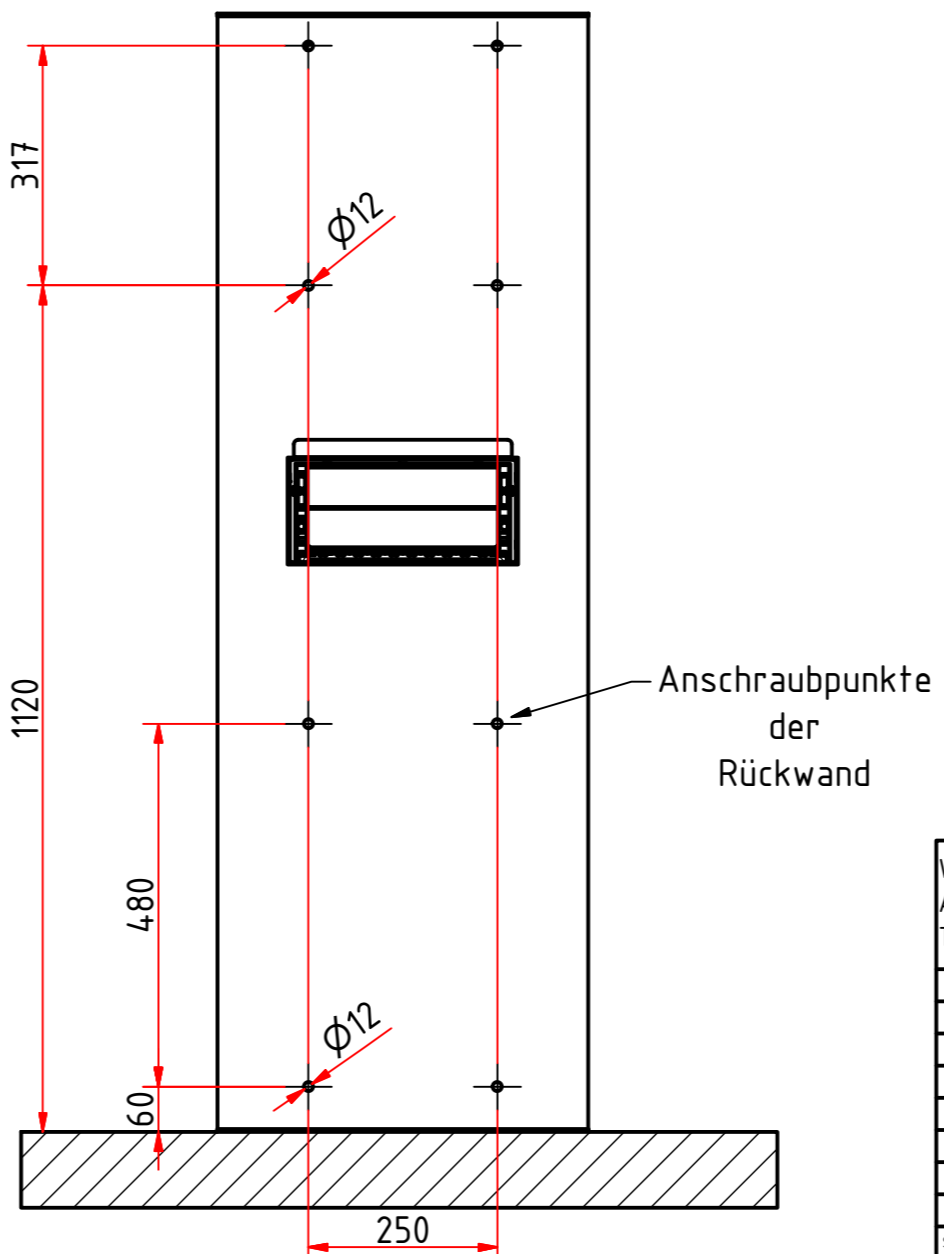
C-C ( 1 : 10 )
