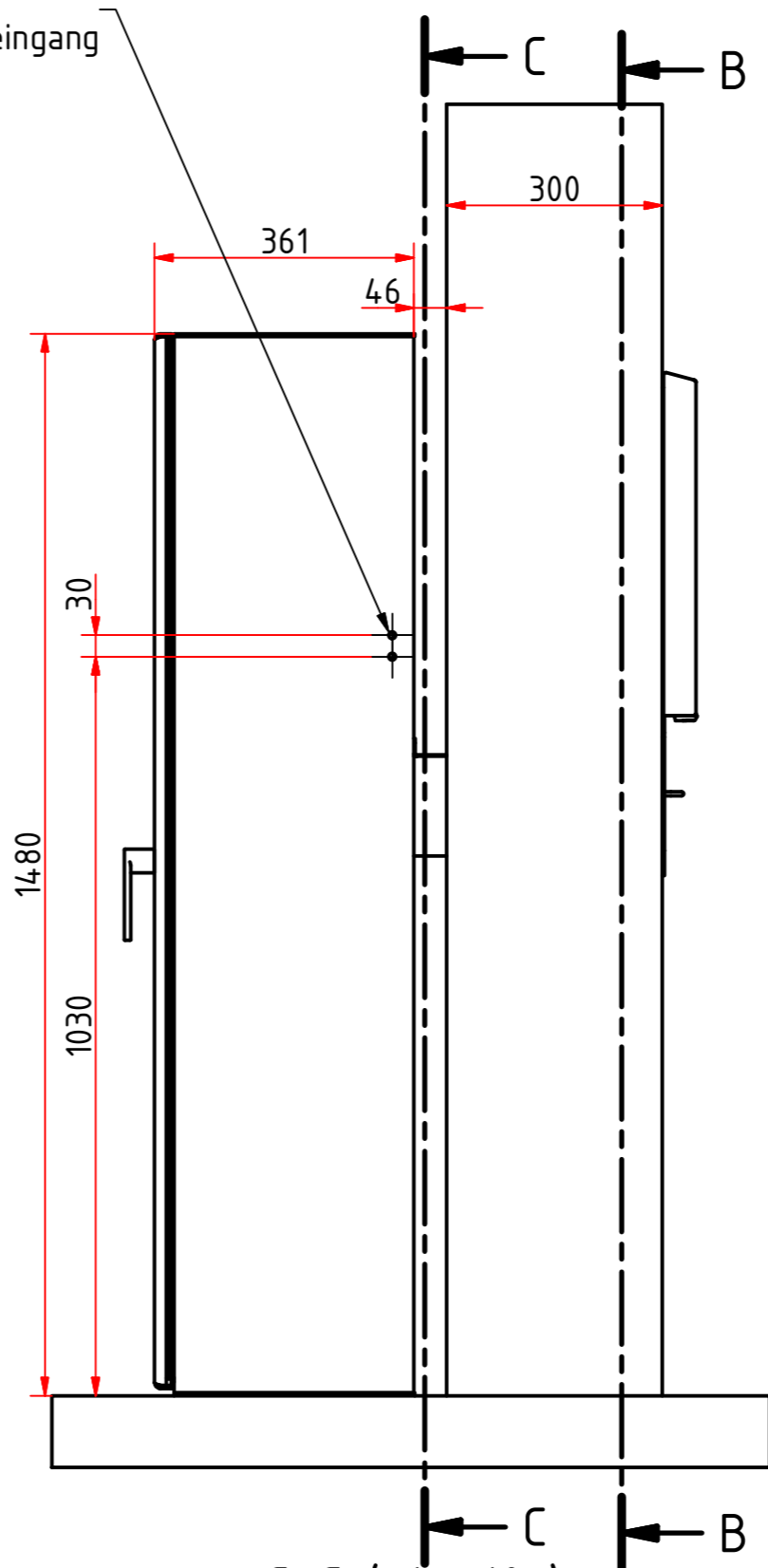
C-C ( 1 : 10 )
