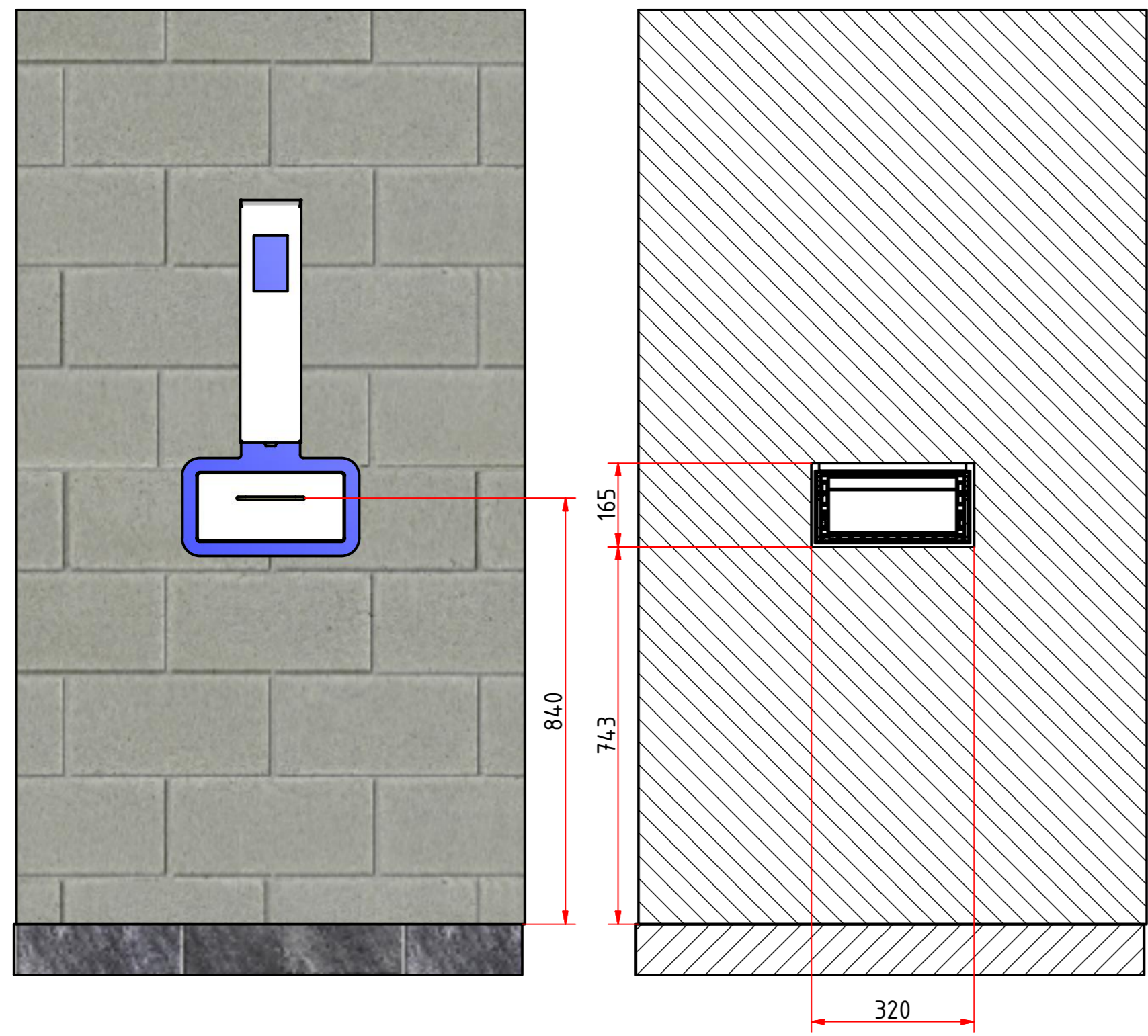
B-B ( 1 : 10 ) Mauerdurchführung
